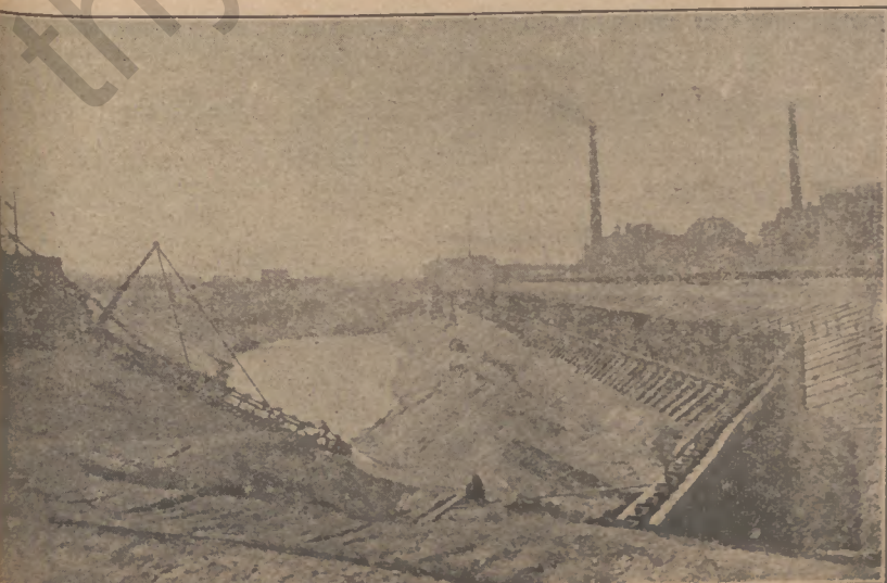
Baugrube für die zweite Abfliegelschleuse des Rhein-Herne-Kanals in Duisburg. Bild III: Nach der Wasserabsenkung.
