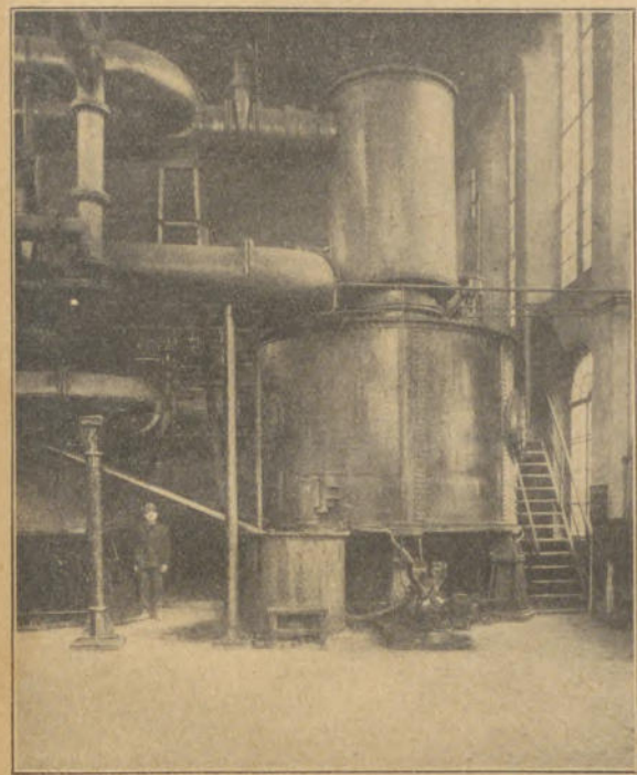
Ammoniak-Sättiger.
