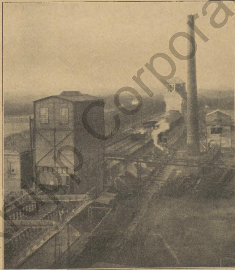
Roksofenanlage der Abteilung Hoerder Verein.
