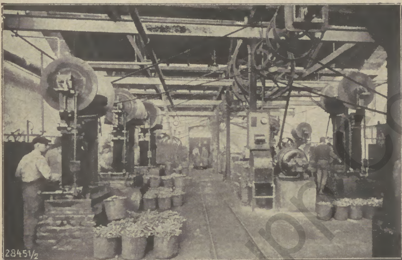
Bild 2: Friktionspressen
