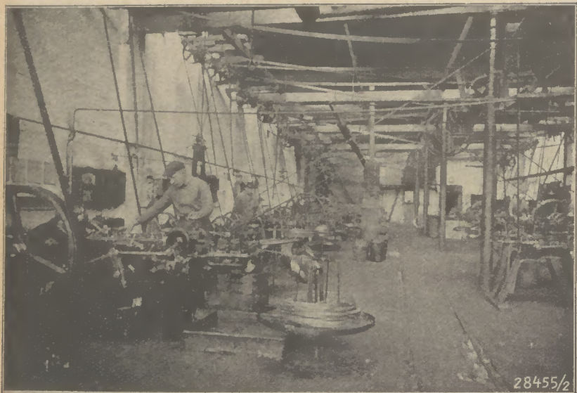
Bild 5: Kaltpressen. — Vorn rechts eine kleine Schlagpresse mit Brettfedern
