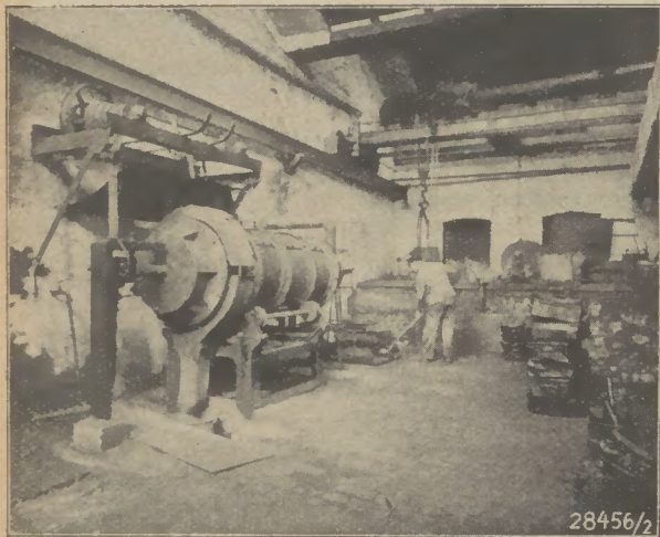
Bild 6: Rotierende Glühmaschine
