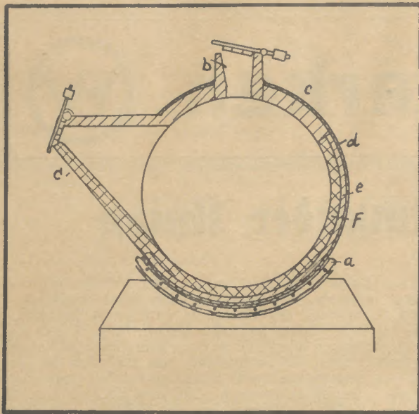
Abb. 2: Rollmischer
