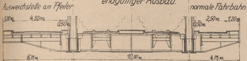
Abb. 3: Brückenquerschnitt.
