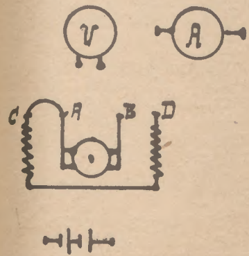
Mischhaltung der Gleichstrommaschine
