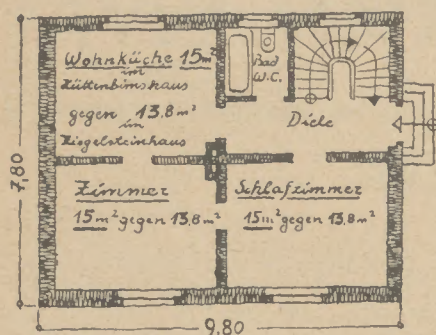
Bild 3: Kleines Einfamilienhaus in Leichtbeton aus Union-Hüttenbims Grundriss des Erdgeschosses
