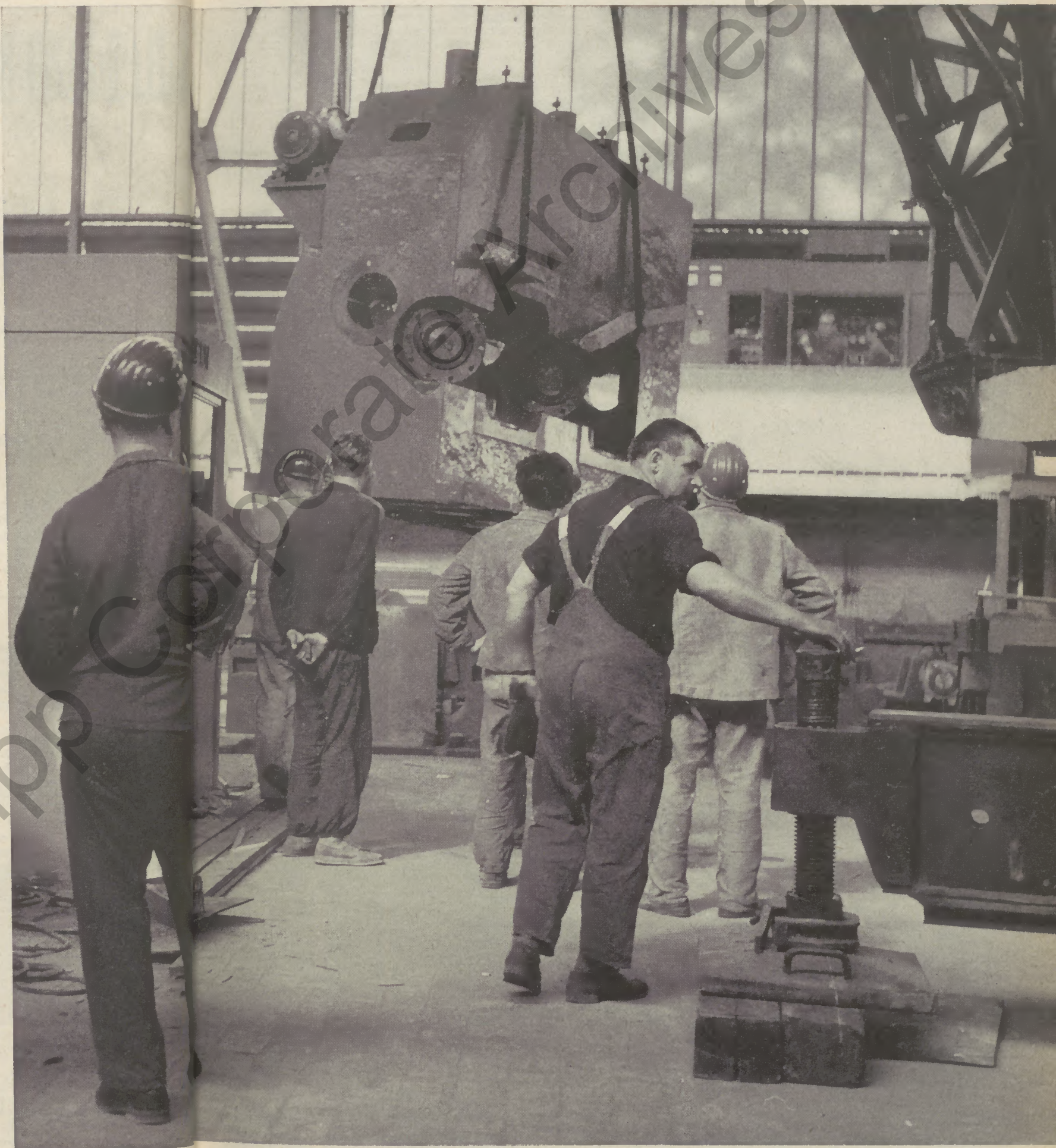
Die Rohrwarmzieherei 4 im Aufbau. Das Lösewalzwerk wird montiert. Am 10. Dezember 1963 drückte Direktor Goedecke auf den Startknopf. Nach Überwindung der üblichen Kinderkrankheiten werden seit Mitte Januar etwa 1 000 Rohre pro Schicht gezogen. Das Ziel liegt bei 1 500 im Durchschnitt. Zum Unterschied gegen die RZ 3 können Wandstärken bis herunter zu 2 1/2 mm und Längen bis 11 m erreicht werden.
