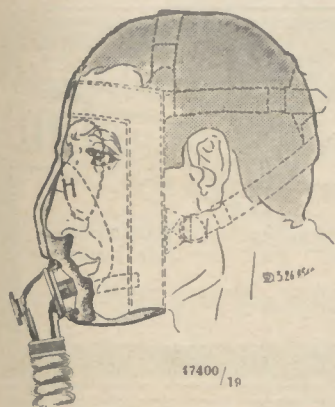
Abb. 9: Schnitt einer Maske mit innerer Hilfsmaske
