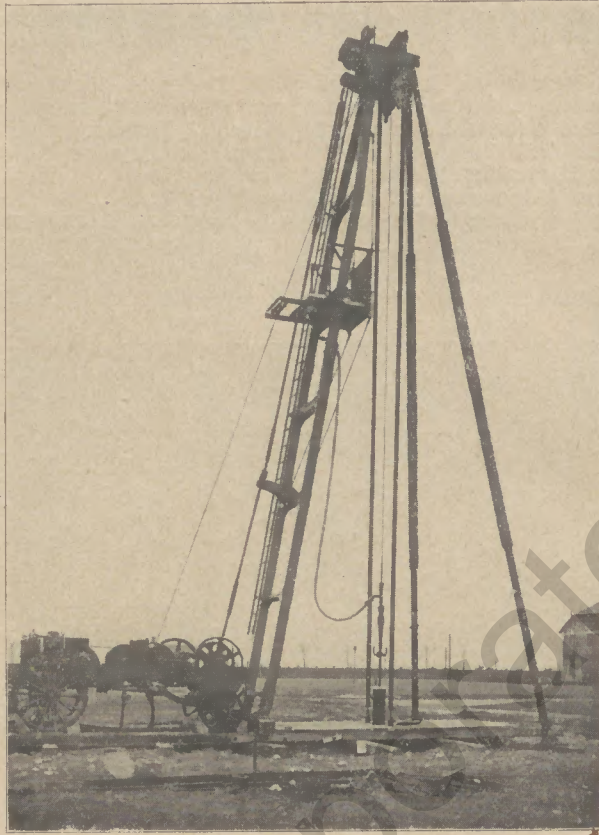
Gesamtansicht einer Bohranlage
