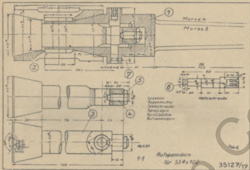
Bild 13: Facharbeit für Dreher: Aufspanndorn, Aufgabe
