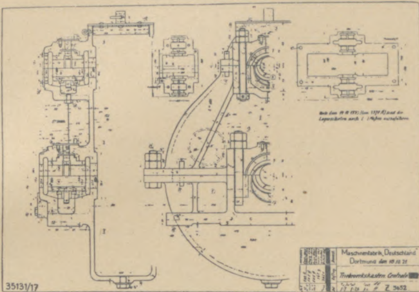
Bild 17: Facharbeit für Formner: Triebwerkstasten, Aufgabe
