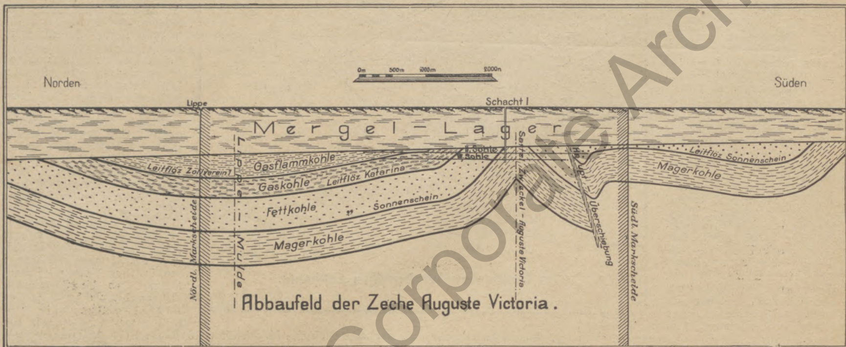
Profil durch das Abbaufeld der Gewerkschaft Auguste Victoria.
