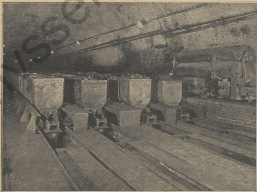
Füllort am Schacht 1 auf der 3. Sohle der Zeche Auguste Viktoria.
