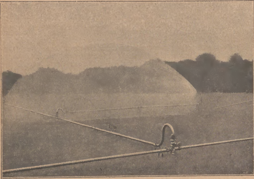
„Phönix“-Weitstrahl-Feldregner (für Großfelder).
