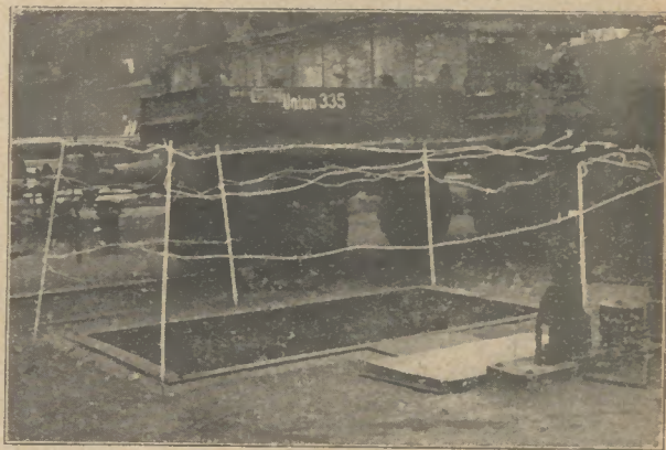
Bild 5: Bessere Kenntlichmachung einer Baugrube im Freien durch weißen Anstrich
