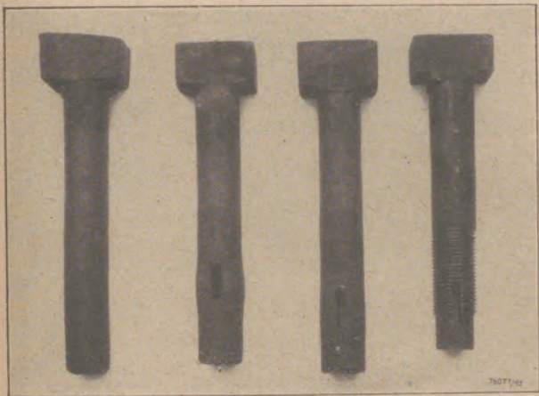
Abb. 2: Freiformschmiede Werdegang einer Ständerfußschraube
