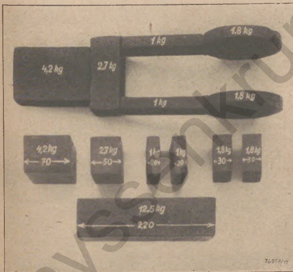
Abb. 3: Freiformschmiede Gabelstück (Inhalts- und Gewichtsrechnung)
