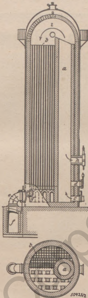
Abb. 7. Winderhitzer nach Cowper
