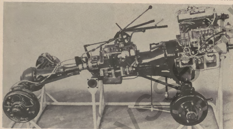
Ein betriebsfertiges — hier nur zur Verdeutlichung der inneren Vorgänge aufgeschnittenes — Modell eines neuzeitlichen Automobil-Motors bzw. des Fahrgestells (Foto: Daimler-Benz AG)
