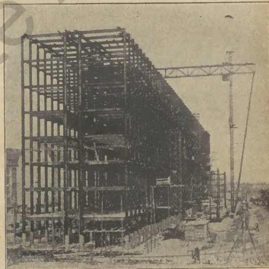
Stahlstelett des Siemens-Hochhauses in Berlin, erbaut von der Brückenbauanstalt der Dortmunder Union
