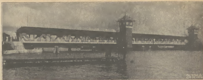
Die doppelstägige Pregel-Drehbrücke in Königsberg (Pr.), erbaut von der Brückenbauanstalt der Dortmunder Union
