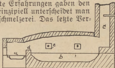
Abb. 6: Puddelofen
