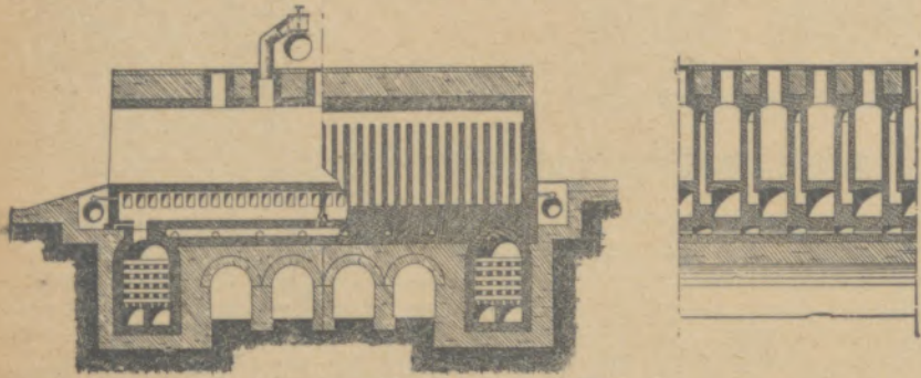
Otto-Hoffmann-Koksöfen.
