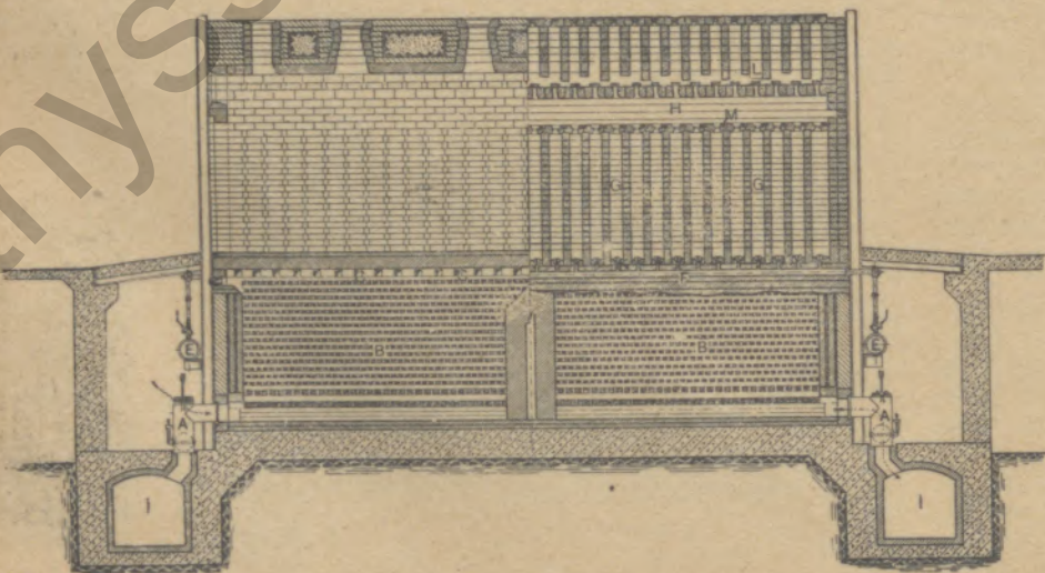
Koppers-Regenerativöfen.
