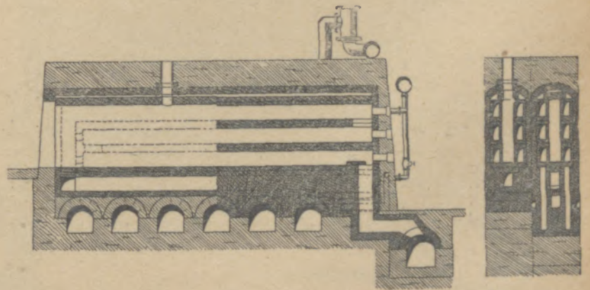
Semet-Solvay-Kokssofen.
