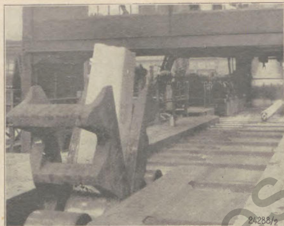
Blockwalzwerk der Hütte Ruhrort-Meiderich
