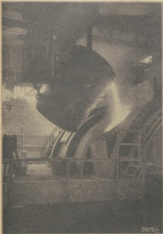
Eingießen von Roheisen in einen Mischer beim Hoerder Verein
