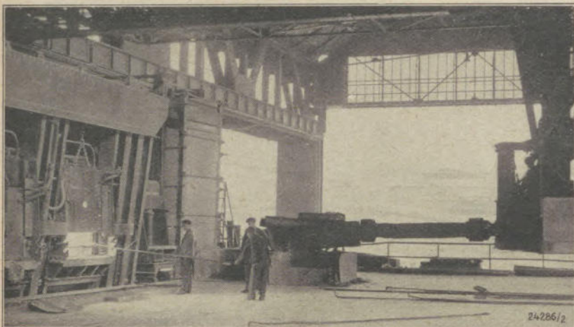
Neuer Talbotofen im Martinstahlwerk der Hütte Ruhrort-Meiderich
