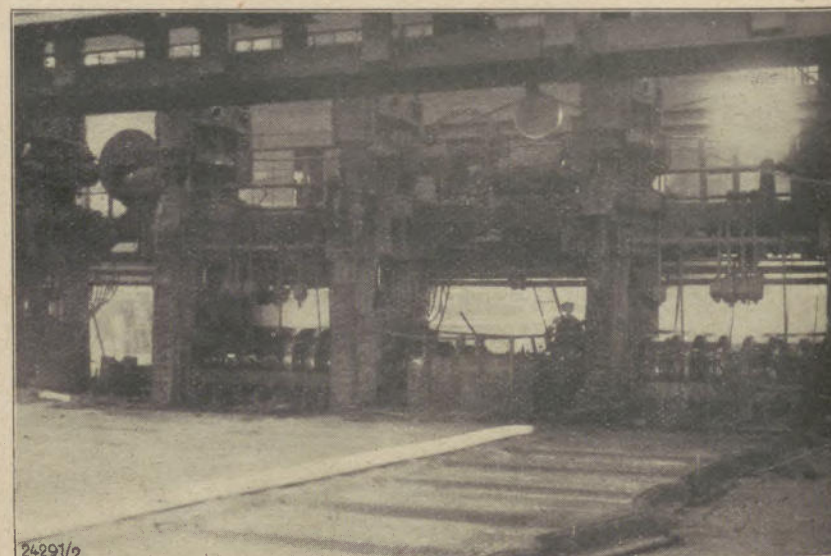
Schwellen-Walzwerk der August Thyssen-Hütte Hamborn
