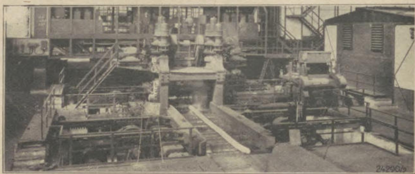
Walzenstraße im neuen Walzwerk IV der Dortmunder Union
