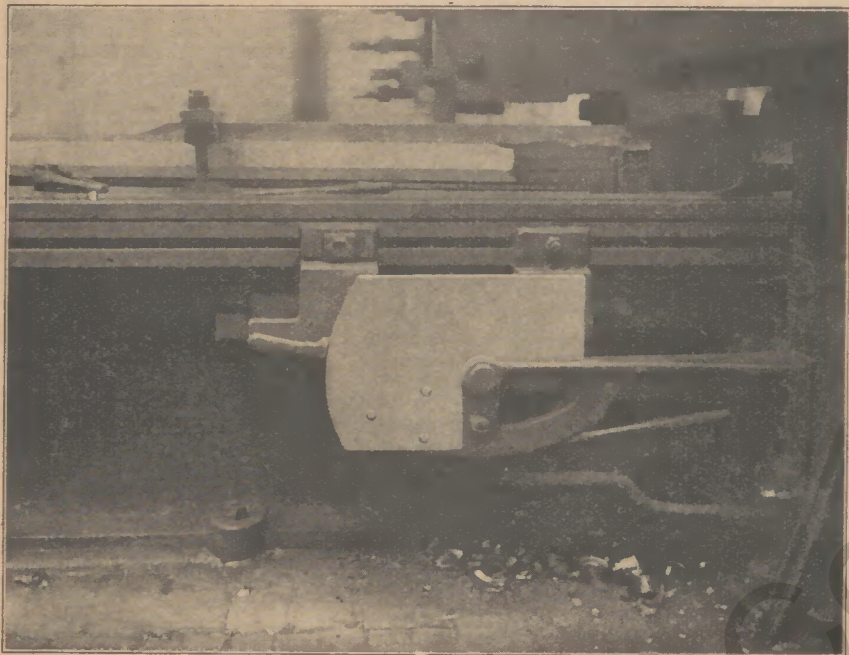
Der den Unfall verursachende Handgriff mit der nunmehr jede Verletzung ausschließenden Schutzverkleidung
