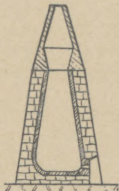
Abb. 4. Stenrischer Stückofen
