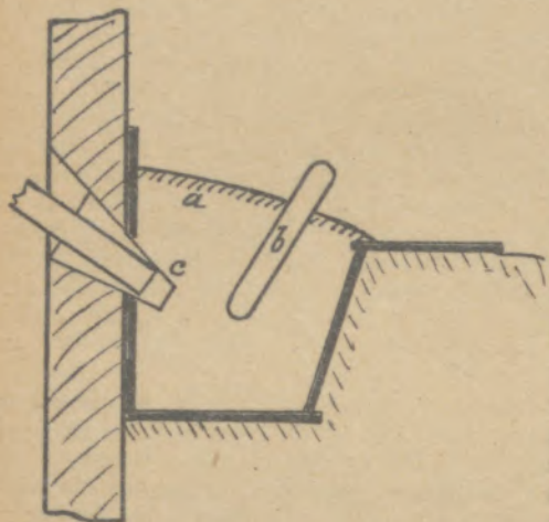
Abb. 6. Frischfeuer (schematisch)
