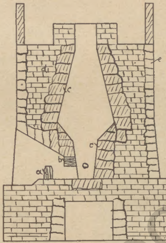
Abb. 3: Hochofen mit offener Brust
