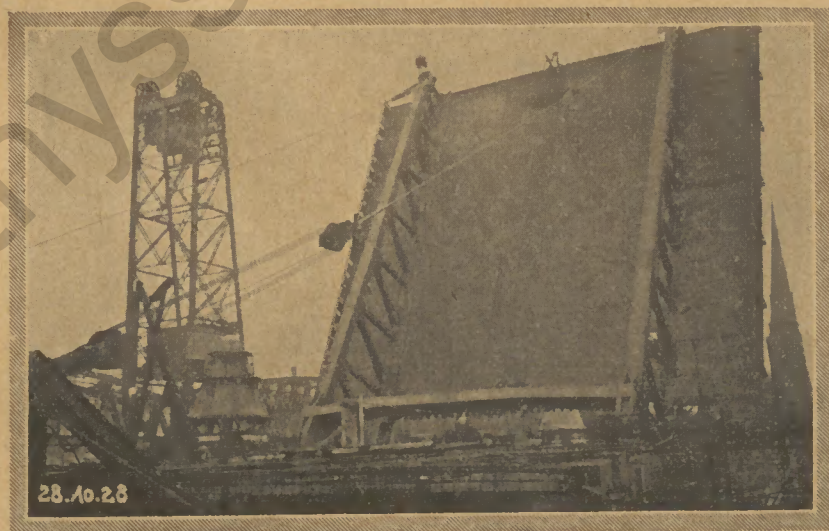
Einbauen der Brücke in den Pfeiler
