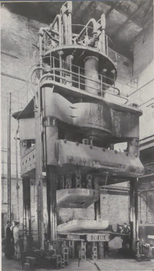
Die lichte Höhe dieser 1000-Tonnen-Kümpelpresse beträgt vier Meter.
