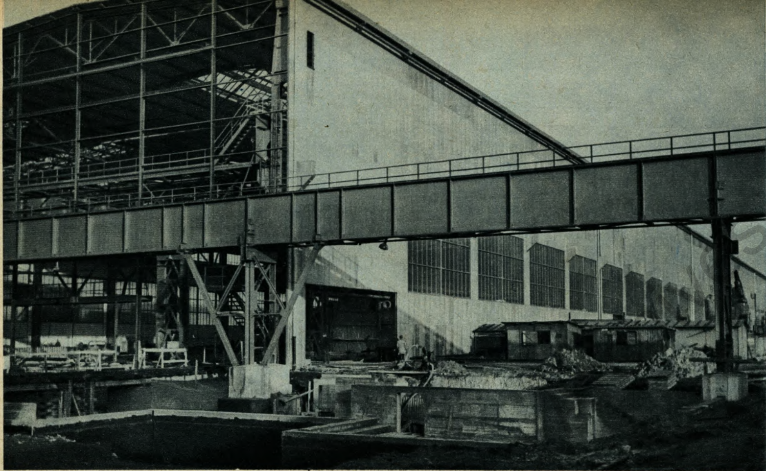
Die Werkshallen für die neue kontinuierliche Halbzeugstraße der Westfalenhütte sind errichtet. An der maschinellen Ausrüstung wird mit Hochdruck gearbeitet, sodaß der Termin der Inbetriebnahme gehalten werden kann
