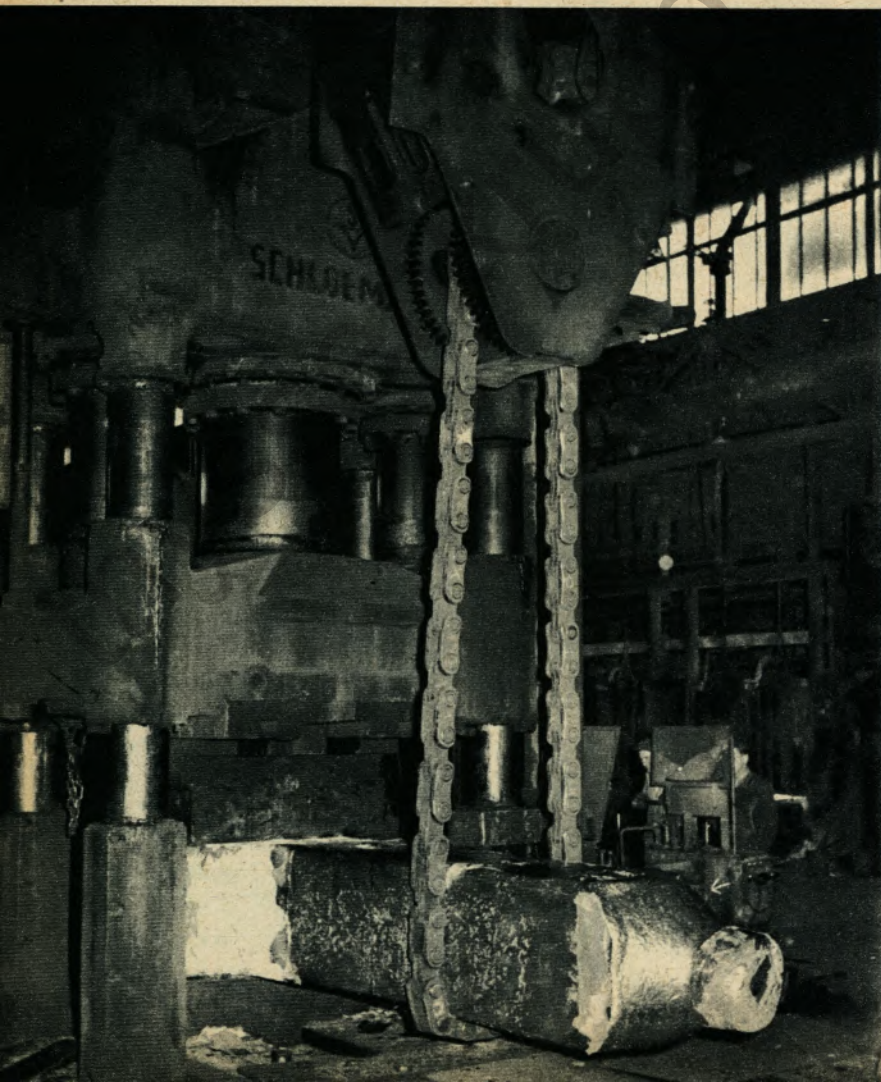
Unter dem wuchtigen Hammer werden die großen Wellen rohggeschmiedet
