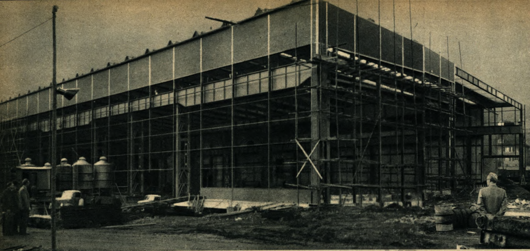
In dieser neuen Halle der Hohenlimburger Walzwerke wird die kontinuierliche Mittelbandstraße errichtet, die gleichzeitig mit der Halbzeugstraße der Westfalenhütte in Betrieb gehen soll
