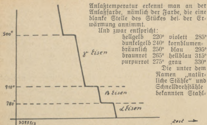
Abb. 5: Temperaturverlauf beim Abkühlen von reinem Eisen
