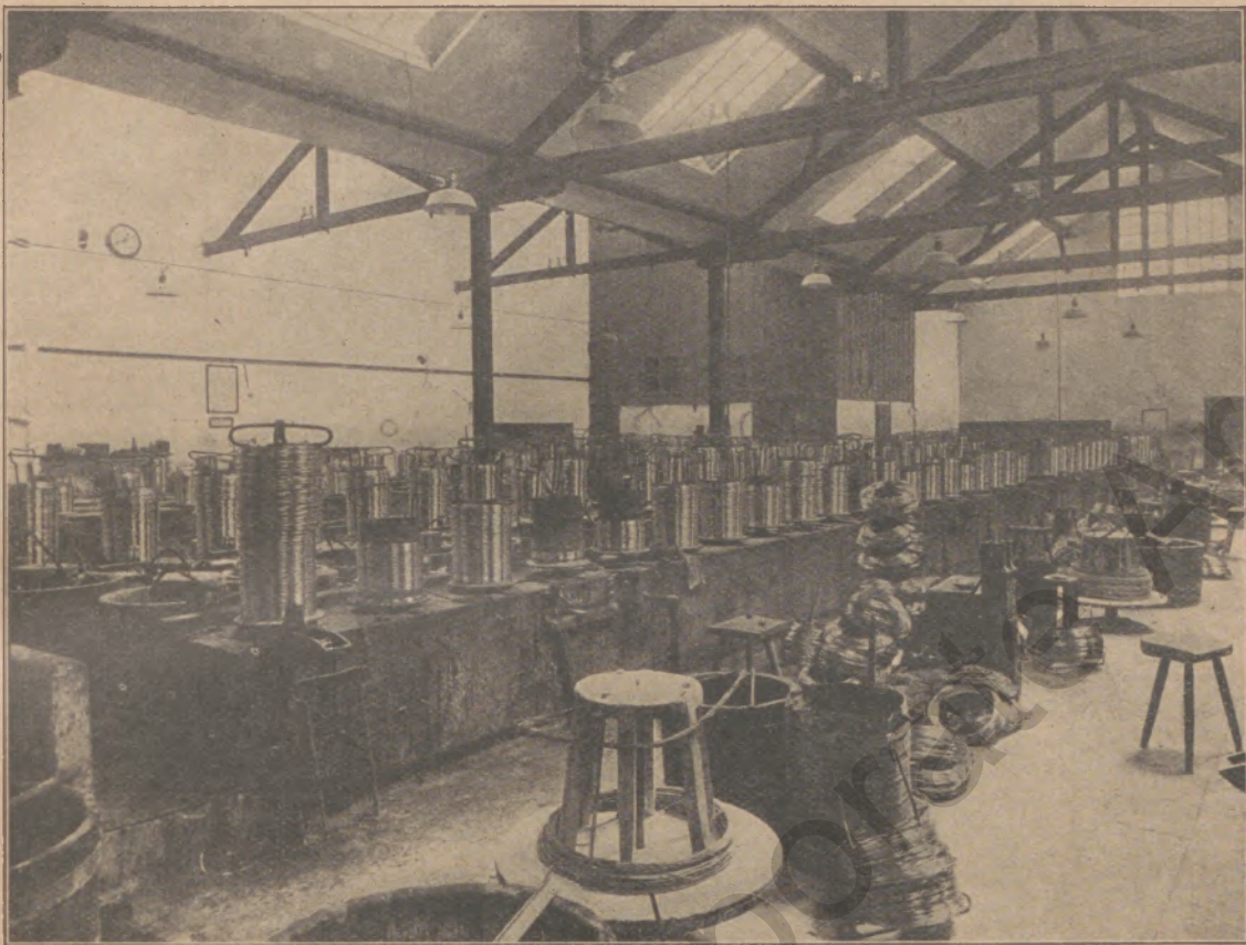
Inneres der Drahtfeinzieherei der Firma Gebrüder Knipping, Altena Man sieht, wie sich Scheibe an Scheibe reiht und die Verfeinerung im großen Stile durchgeführt wird (Zum untenstehenden Aufsatz)
