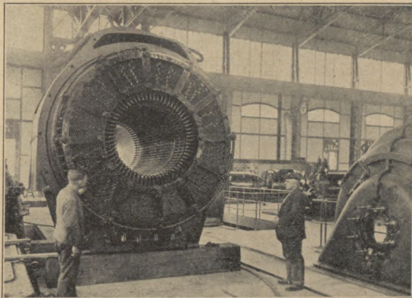
Der Stator des neuen Turbo-Generators. Seine Dimensionen werden durch die neben ihm stehenden Monteure ersichtlich.
