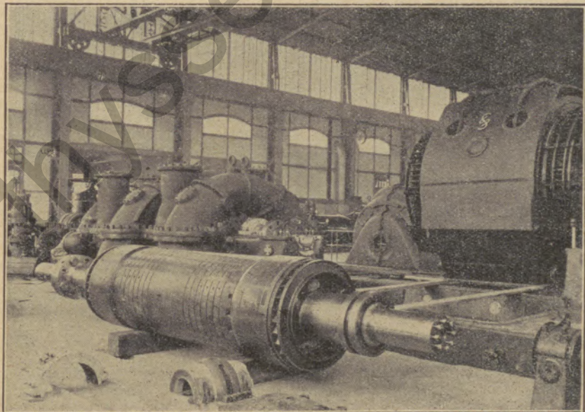
Die Montage des neuen Turbosatzes. Im Vordergrund der Rotor vor dem Einbau.
