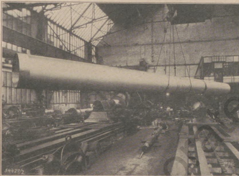
Bild 1: Langes Rohr mit dünner Wandstärke für die chemische Industrie 12 m lang, 835 mm Durchmesser, 17,5 mm Wandstärke, Rohgewicht 42½ t
