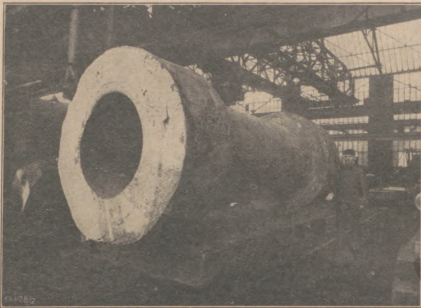
Bild 2: Mantelrohrstück, größter Durchmesser 1570 mm, Länge 3,5 m, auf 850 mm Durchmesser hohlgeschmiedet, Rohgewicht 24 t, aus S. M. Stahl
