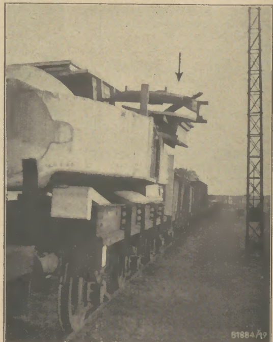
Schlecht beladene Wagen verursachen Eisenbahnunfälle
