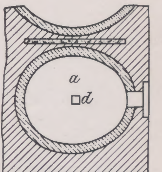
Abb. 3: Englische Bienenforböfen um 1850. Durchmesser etwa 3 Meter, Kuppelhöhe etwa 1 Meter; Beschickung sechs Tonnen Kohle. Verbunden zu Batterien von 30 bis 40 Stück. Garungsdauer 48 Stunden. Ausbringen 55—60 Prozent des Trockenkohleneinlasses
