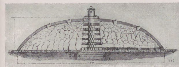
Abb. 1: Steinkohlenmeiler. Dauer eines Werks: 8 bis 14 Tage. Ausbringen etwa 50 Prozent des Trockenkohleneinlasses
