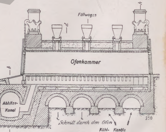
Abb. 8: Coppée-Ofen (Flamm- oder Abhigeofen). Ofenlänge 10,25 Meter, Ofenhöhe 1,70 Meter, Ofenbreite 0,60 Meter, Beschickung 7 bis 8 Tonnen Kohle. Garungszeit etwa 50 Stunden. Ausbringen über 72 Prozent des Trockenkohleneinfasses; Jahresleistung 650/800 Tonnen Koks
