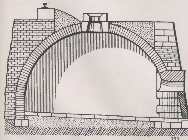
Abb. 2: Durchmesser 2 bis 3 Meter, Höhe 0,7 bis 1,5 Meter, Beschickung 1 bis 2 Tonnen Kohle, Garungszeit etwa 36 Stunden, Ausbringen 50 bis 60 Prozent des Trockenkohleneinlasses
