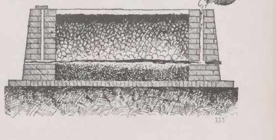
Abb. 7: Schauburger Ofen. Länge des Ofens 8 bis 22 Meter, Höhe des Ofens 1 bis 1,50 Meter, Breite des Ofens 1,50 bis 2,50 Meter; Beschickung bis zu 200 Tonnen möglich. Betriebszeit etwa 6 bis 7 Tage. Ausbringen 50 bis 55 Prozent des Trockenkohleneinfasses. Verringerung der Bedienungsmannschaft je Tonne Koks, niedrigere Reparaturkosten. Geeignet auch zur Verkokung schwach backender Kohle. — Beachte im Mauerwerk rechts und links die Heizkanäle
