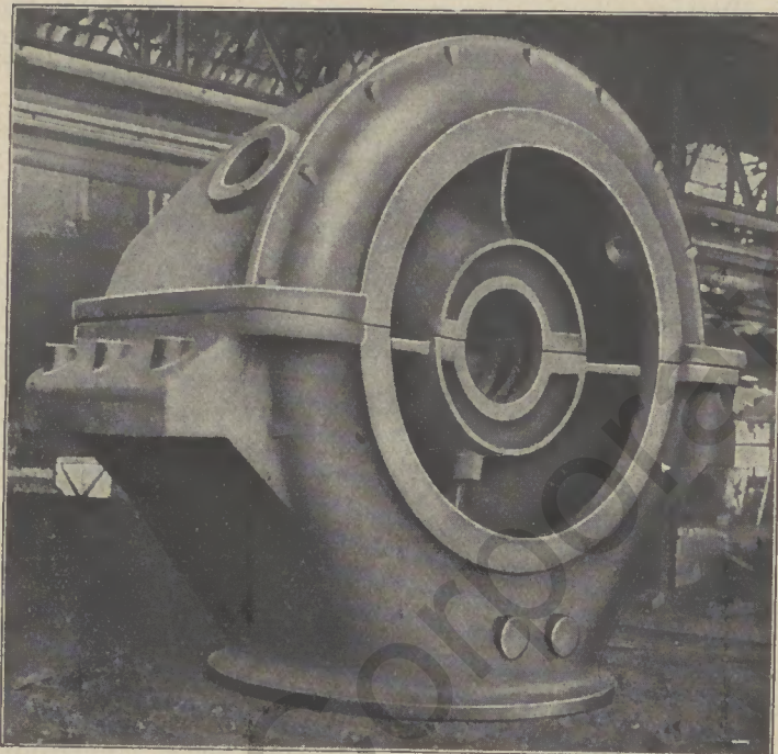
Bild unten: Turbinengehäuse aus Gußeisen von 44 950 kg Gewicht
