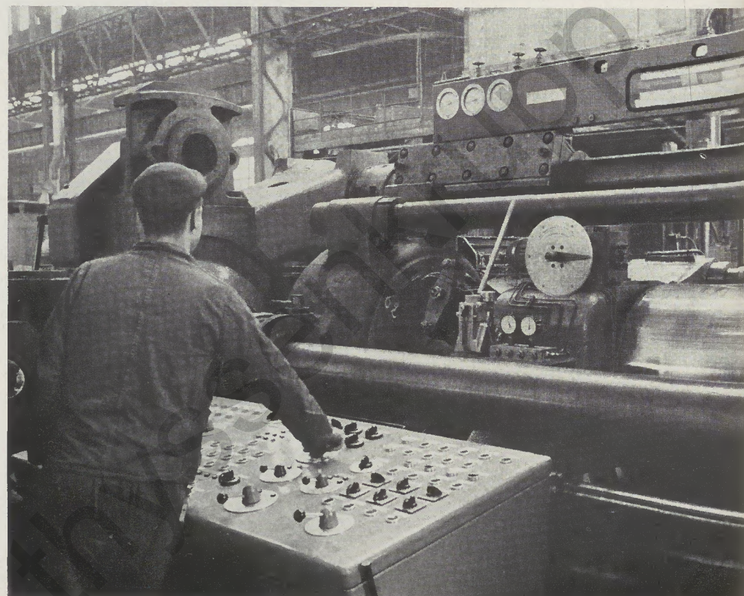
▲ Vor einem Jahr wurde geliefert: eine ölhydraulische Metallrohr- und Strangpresse ▼
