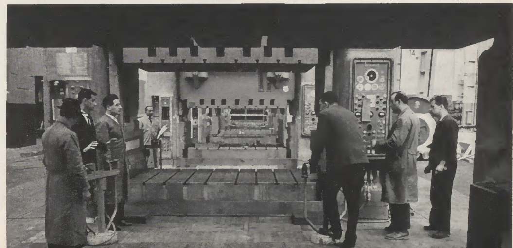
▲ 800-t-Karosseriepresse: Sicherheits-Funktionsprüfung ▼
