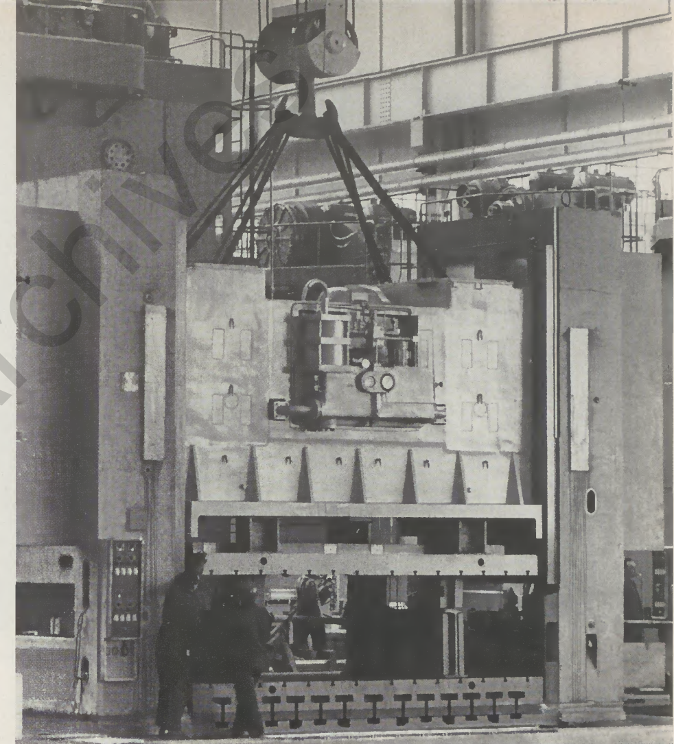
▲ Montage einer 1200-t-Pressen: Einfahren des Stößels
