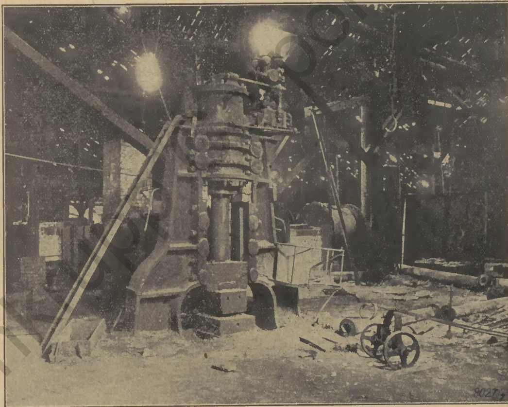
Luppenhammer im Puddelwerk
