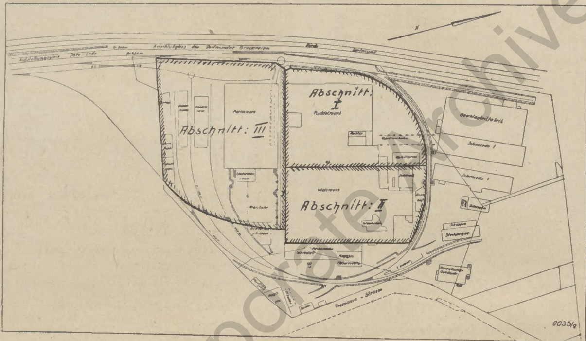
Lageplan des Eisenwerks Rothe Erde. Maßst. 1:1000
