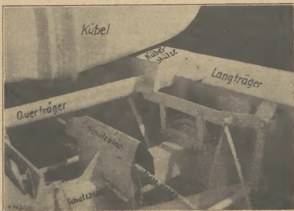
Bild 9: Partie über den Achsen beim Ausstellungswagen
