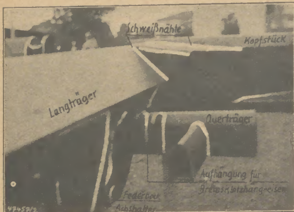
Bild 8: Langträger- und Kopfstücke des Ausstellungswagens
