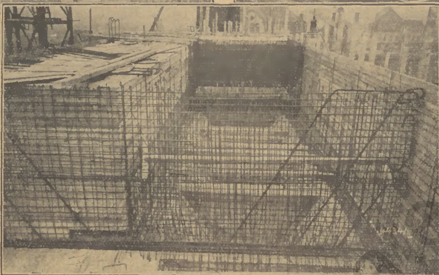
Abb. 7. Armierung der Bunker (Südliche Ansicht)
