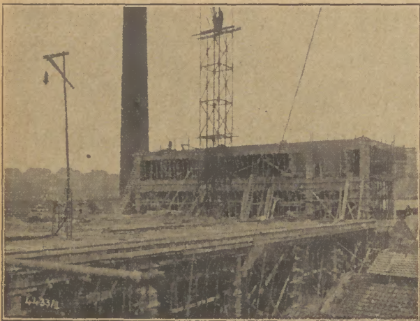
Abb. 6. Bunkeraufbau mit Treppenanlage (Südwestliche Ansicht)
