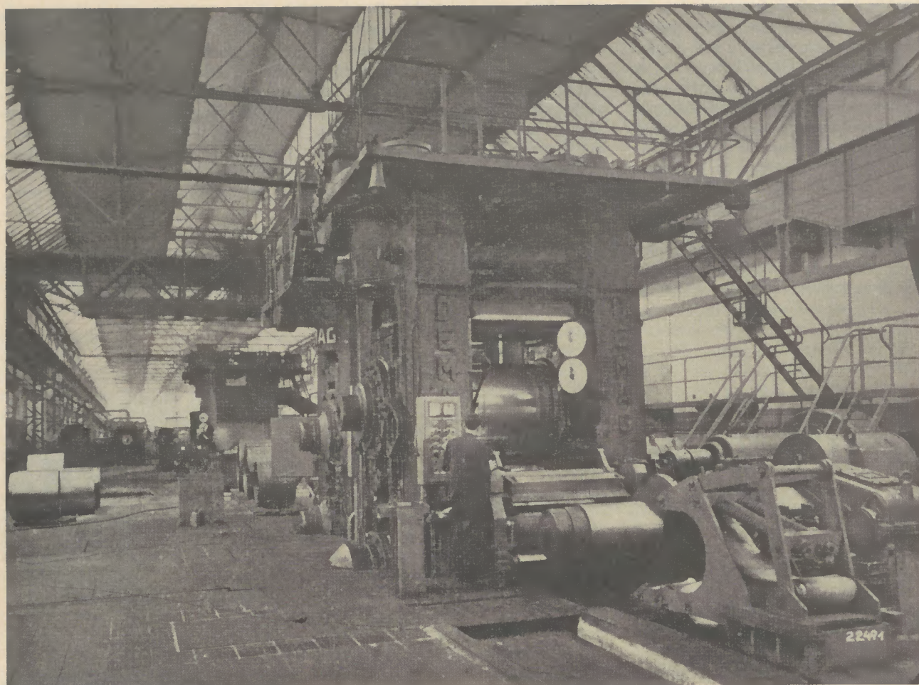
Die neue Dressierstraße im Werk Wissen
