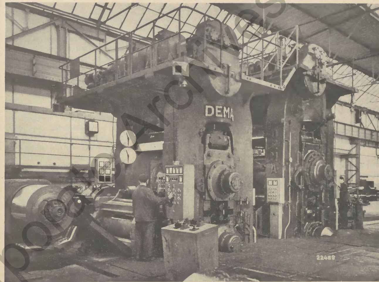
Links das neue Gerüst der Dressierstraße
