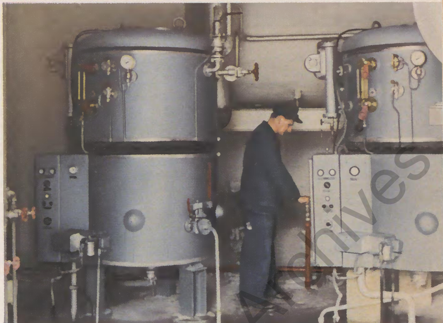
Zwei HK 500 in einem Kunststoff-Werk
