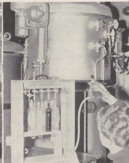
Innenbearbeitung eines großen Behälters (links). — Orsat-Prüfung am HK-Kessel: die Verbrennungsanalyse zur Bestimmung des Kohlenstoffgehalts im Abgasschornstein wird vorgenommen (rechts). Foto rechts: Kurt Fielitz
