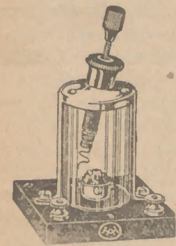
Abb. 2. Der Detektor.
