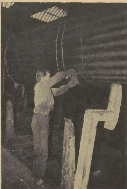
Das Paket in den hinter dem Kühlbett liegenden Sammelaschen ist gefüllt. Auf dem Kühlbett muß zwischen den Rohren ein Abstand geschaffen werden, der es erlaubt, das volle Paket mit Seilen aus den Taschen herauszuheben.
