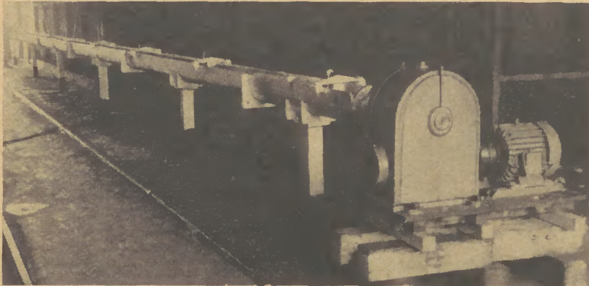
Hier die Schlackentransportschnecke kurz vor ihrem Einbau unter der Walzenstraße. Fotos: Heinz Müller
