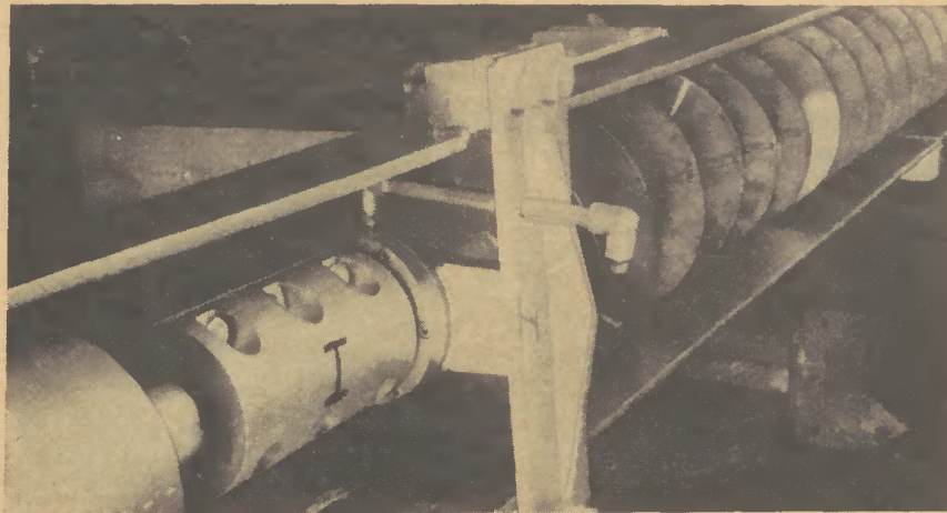
Die Schlackentransportschnecke arbeitet in der gleichen Art wie eine Wurstmaschine.
