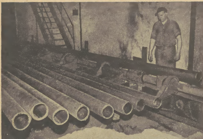
Hier wird gerade ein Rohr durch den Überwurf auf das Kühlbett gelegt. Heinz Zimmermann beobachtet den Vorgang, um eingreifen zu können, wenn es sich nicht richtig einordnet. Aber — wo bleibt eigentlich der Sicherheitshelm auf dem Kopf?
