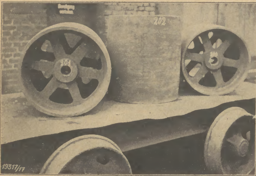
Bild 25: Facharbeit für Lehmformer: Gurttrommel für Transportband (Abguß, gepuht)
