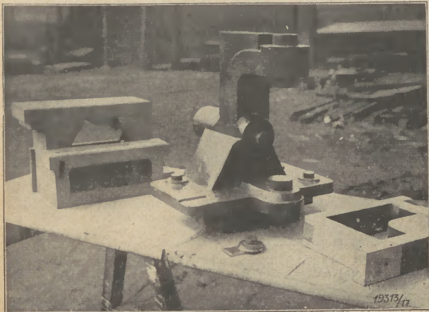
Bild 21: Facharbeit für Modellschreiner und Eisenformer: Weichenbod (Modell und Kernkästen)
