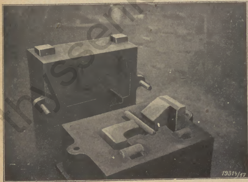
Bild 22: Facharbeit für Eisenformer: Weichenbod (Form mit eingelegten Kernen)
