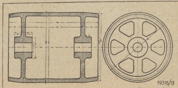
Bild 24: Facharbeit für Lehmformer: Quertrommel (Aufgabe)
