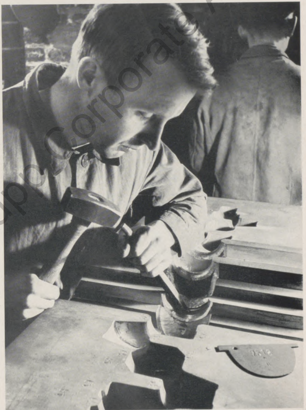
Die letzte Formgebung der Kurbelwellengesenke erfordert ein sauberes Arbeiten nach der Schablone; Werk Remscheid
