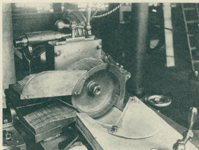
Die Nadelspitzen werden geschliffen.
