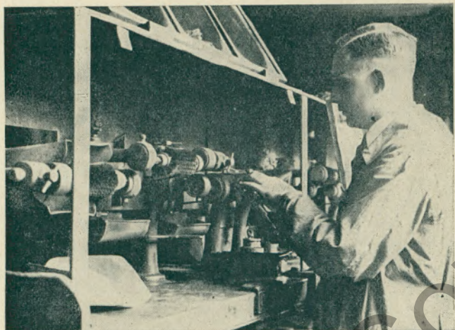
In der Krazmaschine werden die rauen Nadeln geglättet
