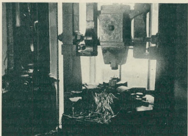
Die Stellen für das Nadelöhr werden vorgestanzt.
