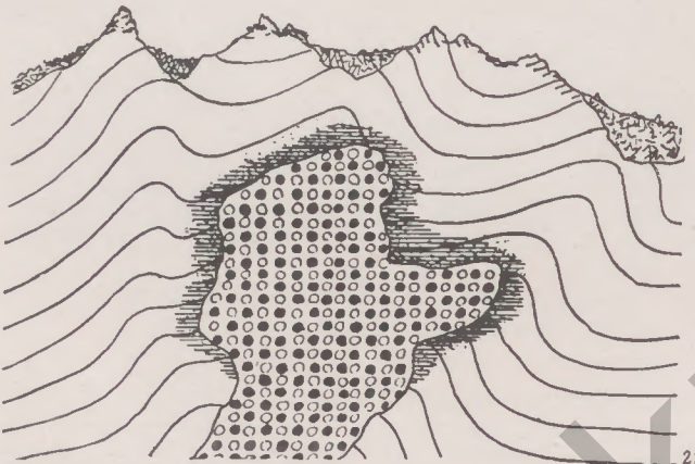
Bild 5: Der aus dem Erdinnern aufsteigende Schmelzfluß füllt den Hohlraum aus (Schematische Darstellung)
