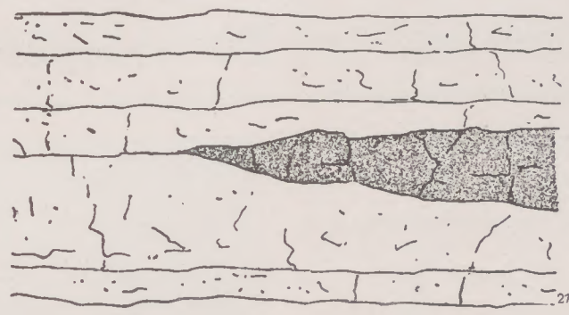
Bild 7: Auskeilender Erzgang
