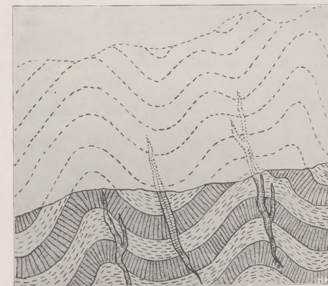
Bild 2: Schema eines Faltengebirges. Durch die Faltung sind Spalten aufgerissen
