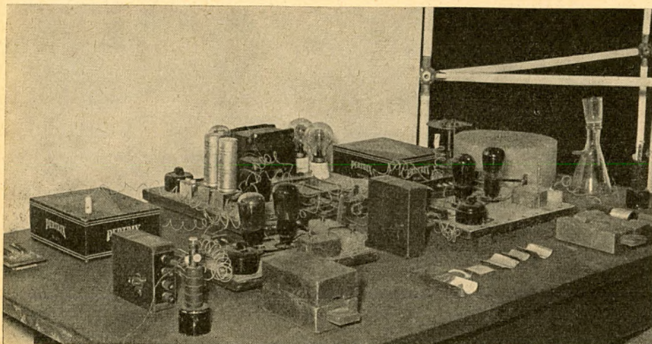
So fing es an: Arbeits-tisch des großen deutschen Pioniers der Atomforschung, Prof. Hahn. Mit dieser Versuchsanordnung hat Prof. Hahn die erste Atomspaltung bewirkt.
