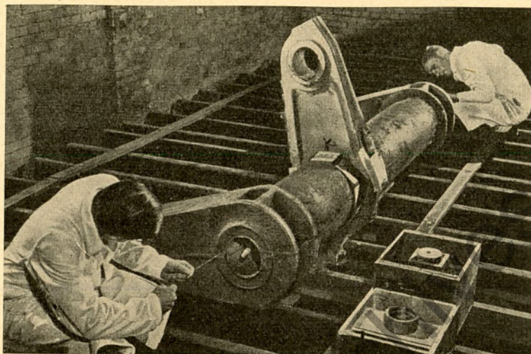
Radioisotope in der Industrie Hier werden Radioisotope zum Durchleuchten eines schweren Gußrohres verwendet. Die Filmplatten liegen oben in der Mitte des zu prüfenden Maschinenteiles.
