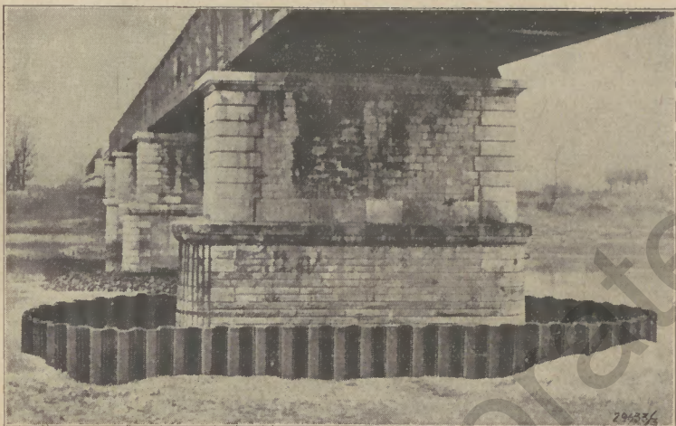
Sicherung einer Seibrücke durch Spundwandisen
