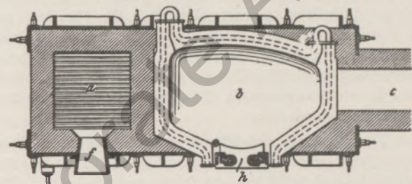
Puddelofen.
