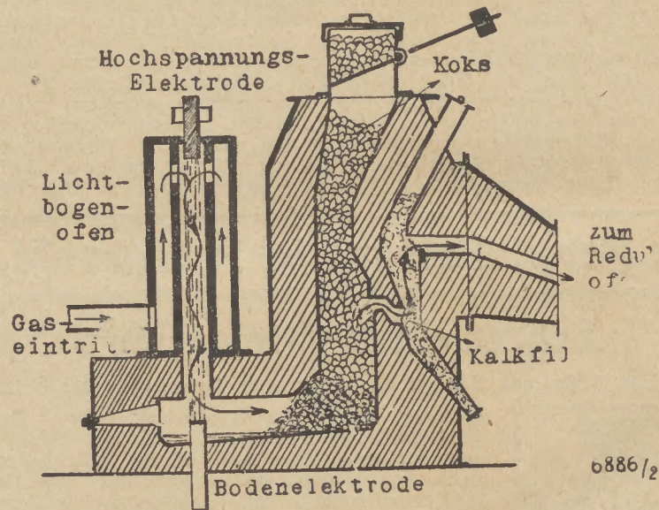
Abb. 2. Hochspannungsflammofen mit Koksgenerator und Kalkfilter
