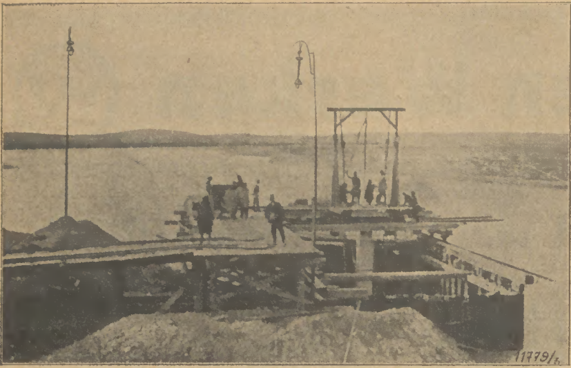
Gründung der Brückenpfeiler für die Euphratbrücke der Bagdadbahn
