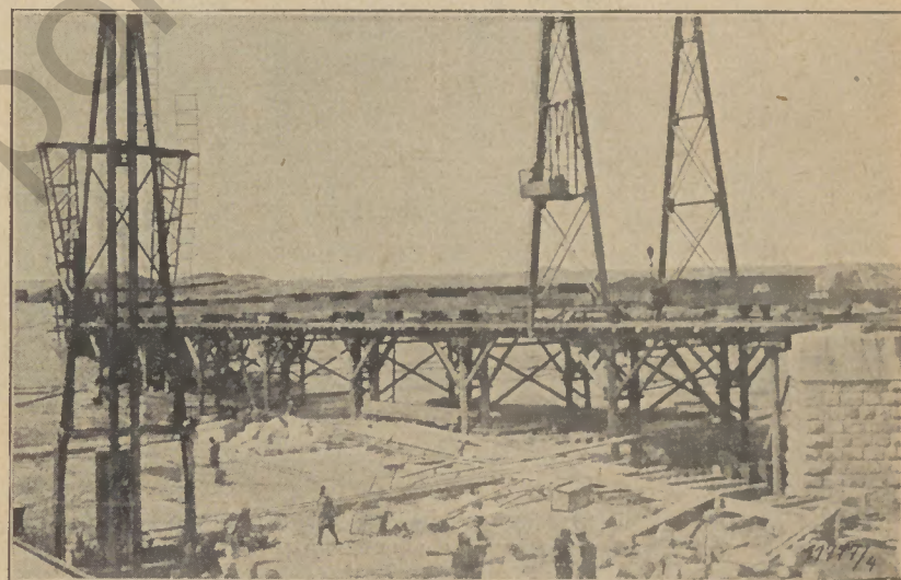
Beginn der Aufstellung der Eisenkonstruktion der ersten Öffnung (Aufgenommen am 6. April 1914)
