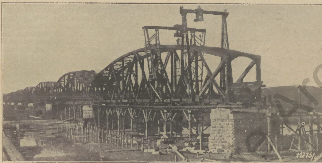
Stand der Aufstellungsarbeiten am 6. Januar 1915
