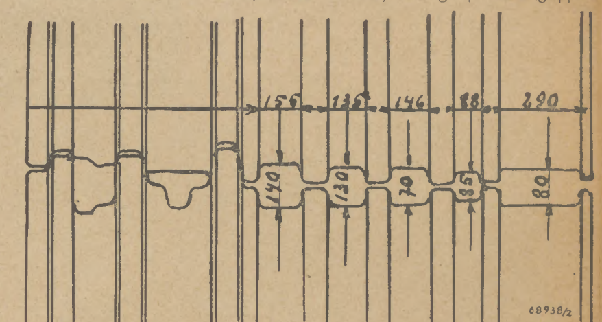
Beispiel einer Walzenzeichnung
